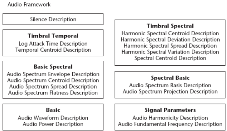
Fig. 3. Audio MPEG-7 descriptors
